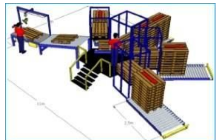
Sortierbühne
